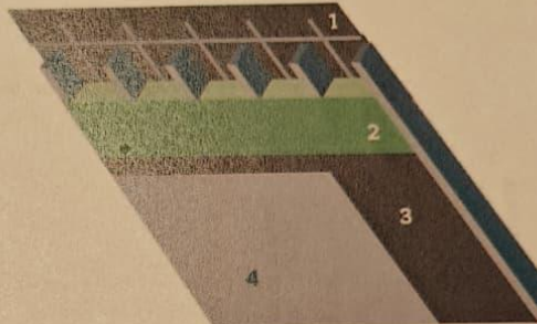
1. Onderdak | 2. Isolatie | 3. Dampscherm | 4. binnenafwerking
